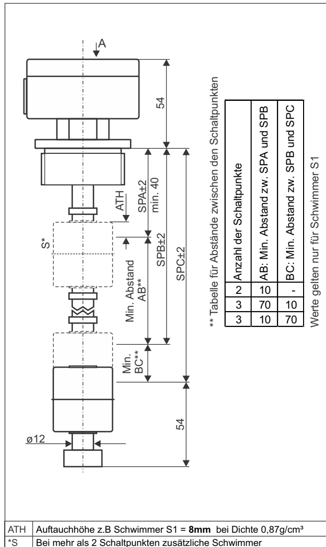
Ansicht A
