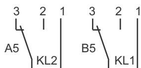
2x Wechsler + Temperaturfühler Beispiel Bestellschlüssel: SSM.2.A5.B5.50.85.7.S1.PT100
