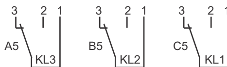
3x Wechsler + Temperaturfühler Beispiel Bestellschlüssel: SSM.3.A5.B5.C5.110.370.850.7.S1.PT100
