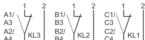
3x Schließer/Öffner + Temperaturfühler Beispiel Bestellschlüssel: SSM.3.A4.B2.C1.90.270.1020.7.S1.PT100
