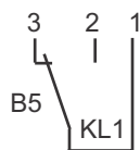
1x Wechsler + Temperaturfühler Beispiel Bestellschlüssel: SSM.1.B5.80.7.S1.PT100
