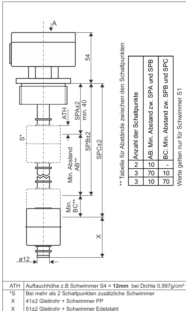
Ansicht A
